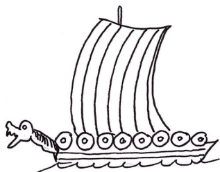
Vikingskib
